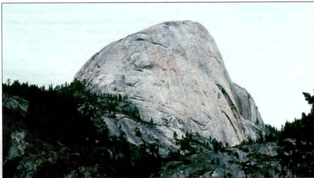
▲ Figura 1.8 El granito es una roca ígnea plutónica especialmente abundante en la corteza continental de la Tierra. A. La erosión ha descubierto esta masa de granito en el Parque Nacional Yosemite de California. B. Muestra de granito que exhibe una textura de grano grueso. (Foto: E. J. Tarbuck.)
