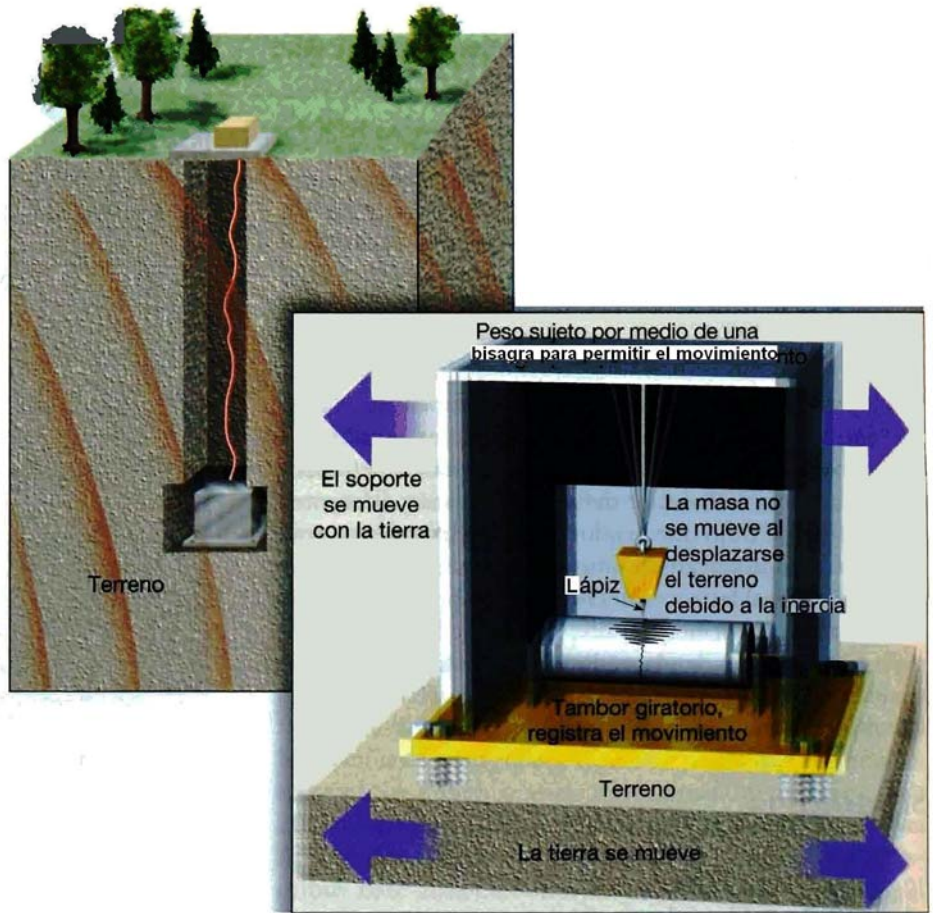
► Figura 11.6 Principio de funcionamiento del sismógrafo. La inercia de la masa suspendida tiende a mantenerla inmóvil, mientras que el tambor de registro, que está anclado al lecho de roca, vibra en respuesta a las ondas sísmicas. Por tanto, la masa estacionaria proporciona un punto de referencia a partir del cual se puede medir la cantidad de desplazamiento que ocurre cuando las ondas sísmicas atraviesan el suelo que está por debajo.
