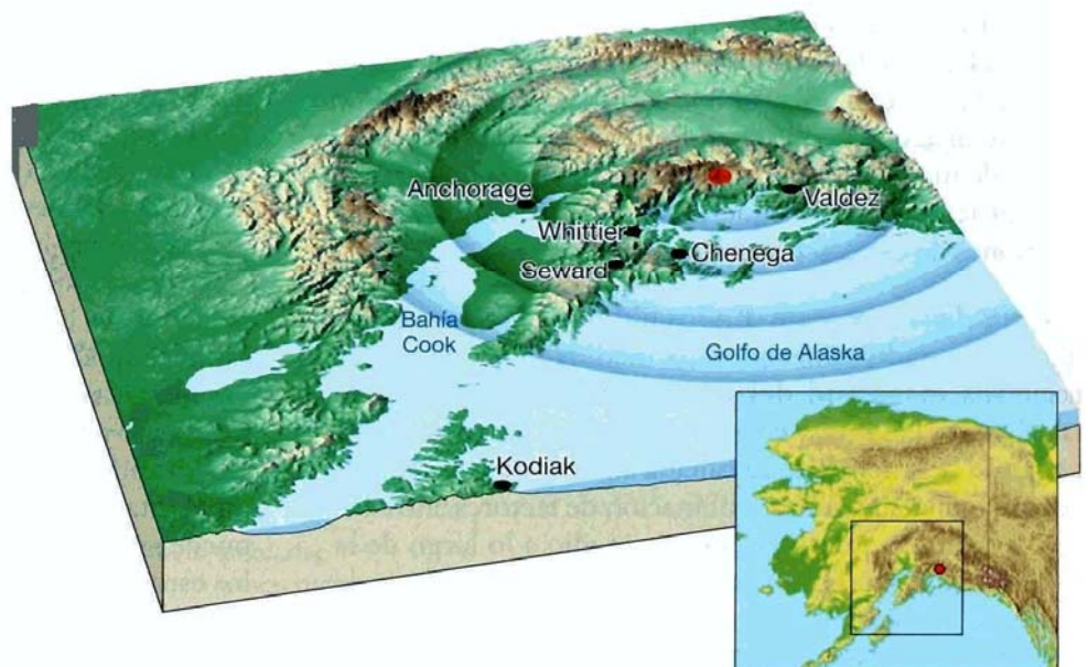
► Figura 11.15 Región más afectada por el terremoto del Viernes Santo de 1964. Obsérvese la localización del epicentro (punto rojo). (Del U. S. Geological Survey.)
