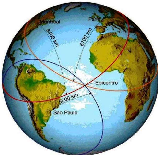
▲ Figura 11.11 El epicentro de un terremoto se localiza utilizando las distancias obtenidas desde tres o más estaciones sísmicas.
