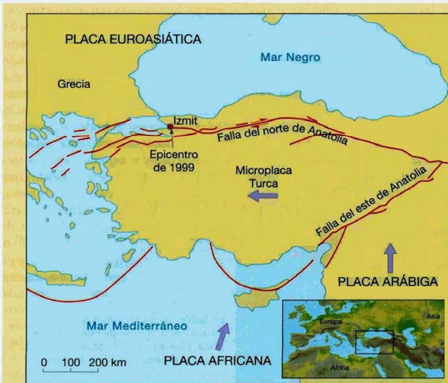
▲ Figura 11.D Los terremotos de Turquía son provocados por el movimiento hacia el norte de las placas Arábica y Africana contra la placa Euroasiática, presionando la pequeña microplaca Turca hacia el oeste. El movimiento tiene cabida a lo largo de dos grandes fallas con desplazamiento horizontal: la falla del norte de Anatolia y la falla del este de Anatolia.
