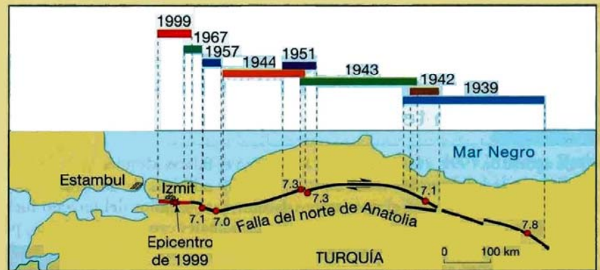
▲ Figura 11.E Este mapa describe la progresión secuencial hacia el oeste de los grandes terremotos a lo largo de la falla del norte de Anatolia entre 1939 y 1999. Se anotan el epicentro y la magnitud de cada uno de ellos. La longitud de cada segmento coloreado indica la extensión de la ruptura superficial a lo largo de la falla para cada acontecimiento.
