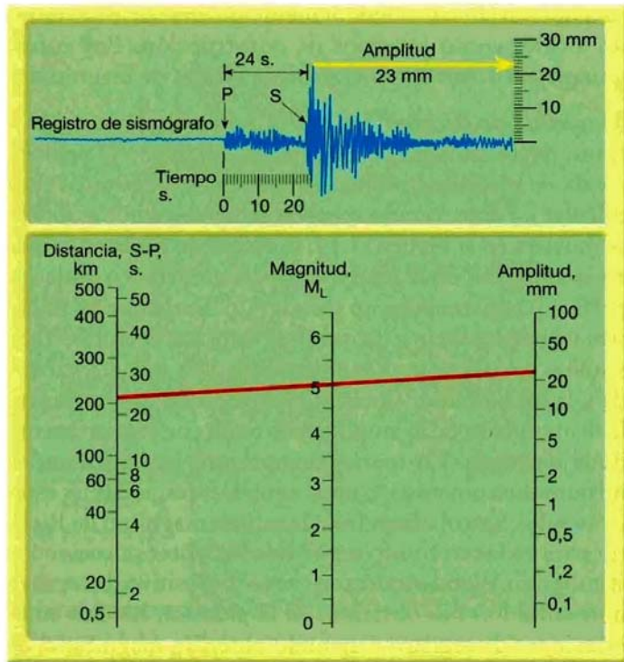
▲ Figura 11.14 Ilustración que muestra cómo puede determinarse gráficamente la magnitud Richter de un terremoto utilizando un registro sismográfico procedente de un instrumento Wood-Anderson. En primer lugar, se mide la altura (amplitud) de la mayor onda en el sismograma (23 mm) y luego la distancia hasta el foco mediante el intervalo de tiempo entre las ondas S y P (24 segundos). A continuación, se dibuja una línea entre la escala de distancia (izquierda) y la escala de amplitud de onda (derecha). Así, deberíamos obtener la magnitud Richter ( M_L ) de 5. (Datos procedentes del instituto de Tecnología de California.)
