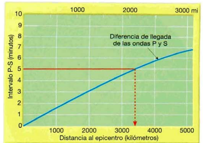
▲ Figura 11.10 La representación distancia-tiempo se utiliza para determinar la distancia al epicentro. La diferencia entre el tiempo de llegada de las primeras ondas P y de las primeras ondas S en el ejemplo es de 5 minutos. Por tanto, el epicentro está aproximadamente a 3.400 kilómetros.
