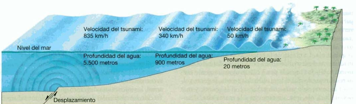
▲ Figura 11.18 Diagrama de un tsunami generado por desplazamiento del suelo oceánico. La velocidad de una ola está relacionada con la profundidad oceánica. Como se muestra, las olas que se mueven en agua profunda avanzan a velocidades que superan los 800 kilómetros por hora. La velocidad disminuye gradualmente hasta 50 kilómetros por hora a profundidades de 20 metros. La disminución de la profundidad reduce la velocidad del movimiento de la ola. A medida que las olas se ralentizan en agua superficial, crecen en altura hasta que se tambalean y se precipitan sobre la costa con tremenda fuerza. El tamaño y el espaciado de este oleaje no están representados a escala.
