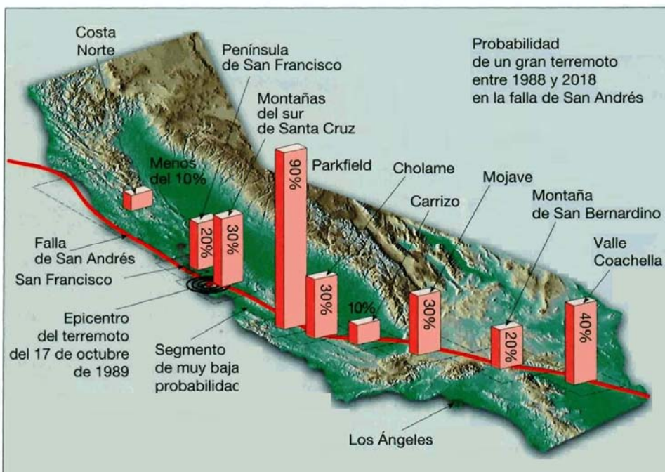
◀ Figura 11.23 Probabilidad de aparición de grandes terremotos entre el año 1988 y el 2018 a lo largo de la falla de San Andrés.
