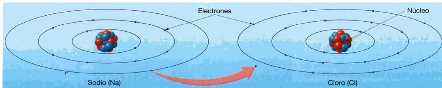
▲ Figura 3.5 Enlace químico de sodio y cloro a través de la transferencia del electrón externo solitario de un átomo de sodio a un átomo de cloro. El resultado es un ion sodio positivo ( \text{Na}^+ ) y un ion cloro negativo ( \text{Cl}^- ). El enlace para producir cloruro sódico ( \text{NaCl} ) se debe a la atracción electrostática entre los iones positivos y negativos. En este proceso, obsérvese que los dos átomos, el sodio y el cloro, han alcanzado la configuración de gas noble estable (ocho electrones en su última capa).
