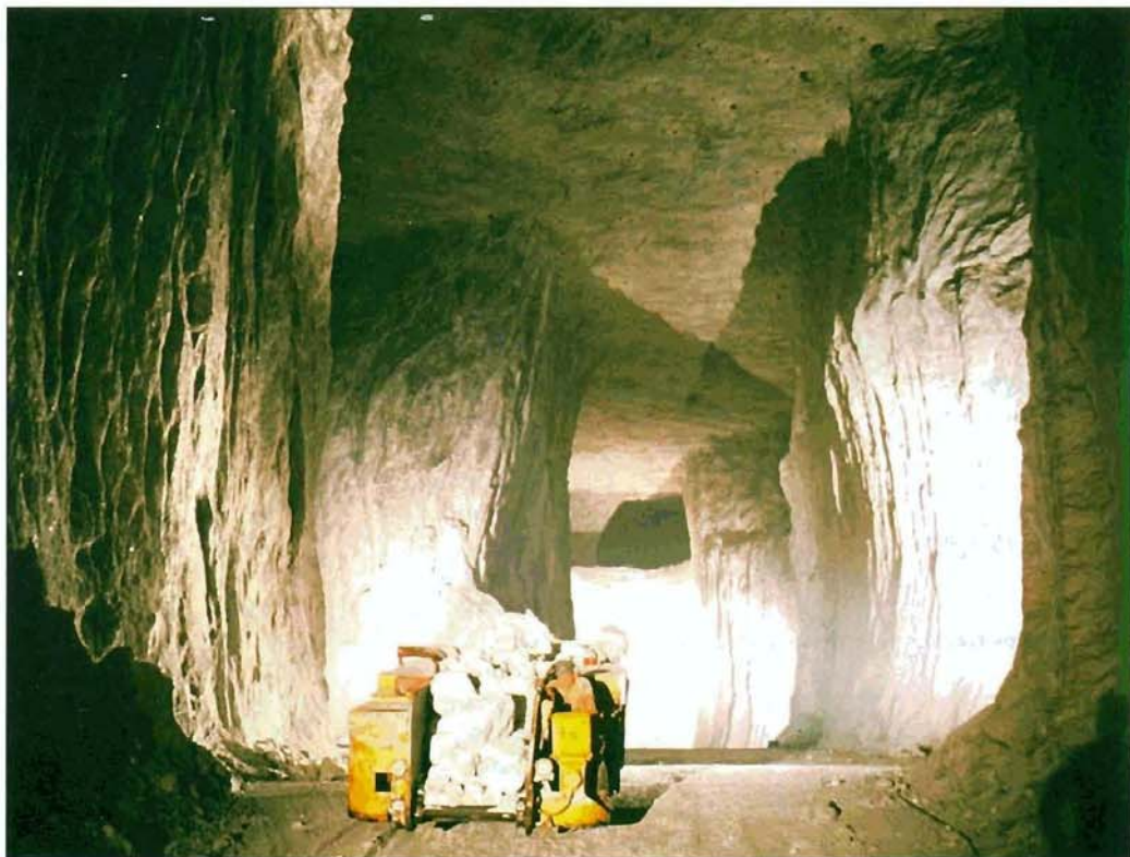
► Figura 3.28 Capa gruesa de halita (sal) en una mina subterránea en Grand Saline, Texas. (Foto de Tom Bochsler.)
