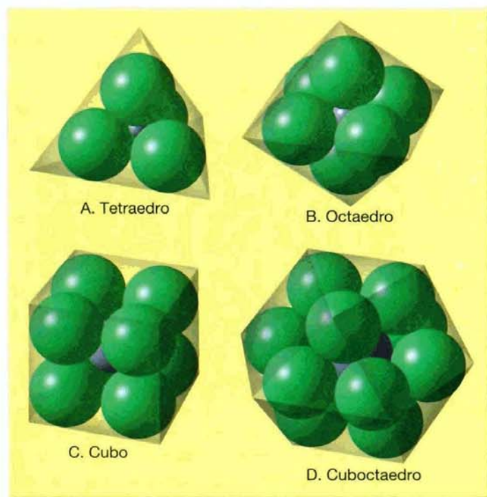
▲ Figura 3.8 Empaquetamiento geométrico ideal para iones positivos y negativos de varios tamaños.
