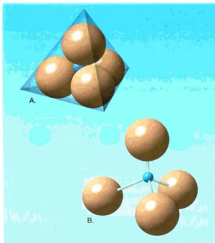
Figura 3.17 Dos representaciones del tetraedro silicio-oxígeno. A. Las cuatro esferas grandes representan los iones oxígeno y la esfera azul representa un ion silicio. Las esferas se dibujan en proporción al radio de los iones. B. Visión extendida del tetraedro utilizando varillas para indicar los enlaces que conectan los iones.
