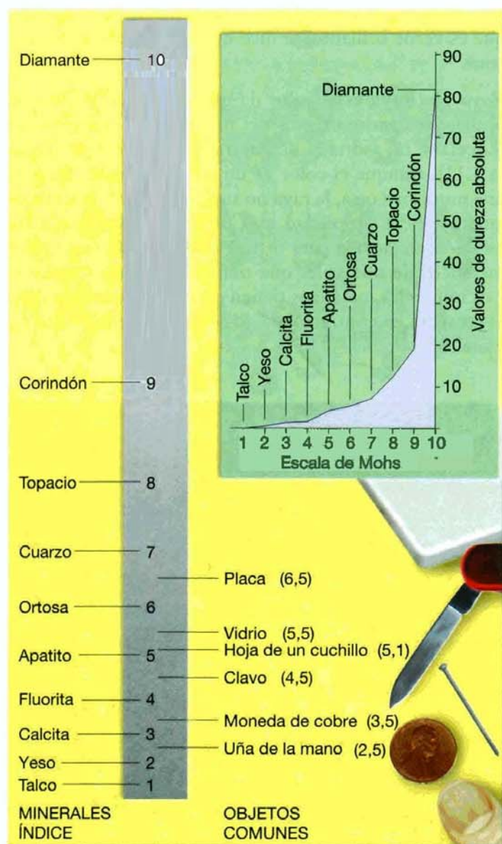
▲ Figura 3.12 Escala de dureza de Mohs, con la dureza de algunos objetos comunes.
