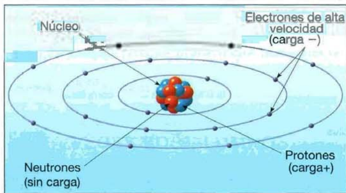
▲ Figura 3.4 Dos modelos del átomo. A. Una visión del átomo muy simplificada, que consiste en un núcleo central, compuesto por protones y neutrones, rodeados por electrones de alta velocidad. B. Otro modelo de los átomos que muestra nubes de electrones de forma esférica (capas de nivel de energía). Obsérvese que estos modelos no están dibujados a escala. Los electrones son de tamaño minúsculo en comparación con los protones y los neutrones, y el espacio relativo entre el núcleo y las capas de electrones es mucho mayor que la mostrada.
