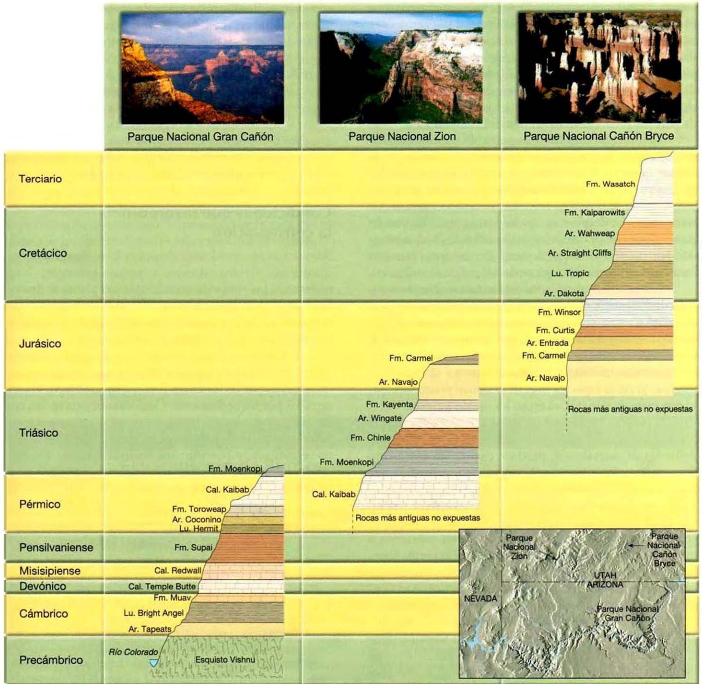
▲ Figura 9.7 La correlación de estratos en tres localidades de la meseta de Colorado revela la extensión total de las rocas sedimentarias en la región. (Tomado del U. S Geological Survey; fotos de E. J. Tarbuck.)
