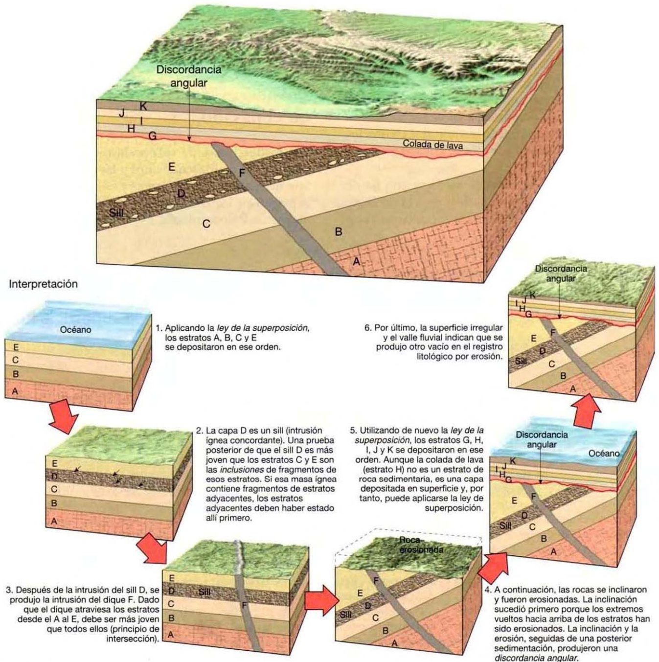
▲ Figura 9.6 Corte geológico de una región hipotética.
